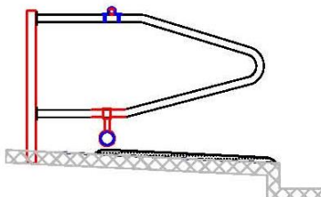
Lejebegrænser med 110 ell 90 mm. rør Monteret med justerbar beslag
