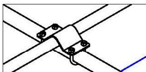
Montering af standard 1½" nakkerør
