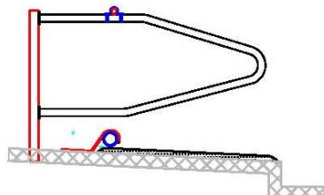
Lejebegrænser med 110 ell 90 mm. rør Monteret med fast bøjlebeslag
