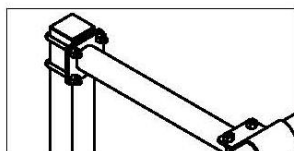
Montering af sengebøjler direkte på 70 X 70 stolpe
