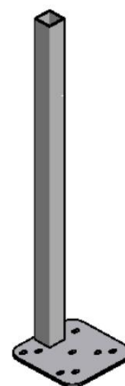
Stolpe 90 x 90 x 4 mm med fodplade - side længde 300 cm 691299-01
