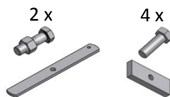
691266 2" 2 x 4 x mont.sæt inkl. 2 stk. fladjern, fladj.møtrik og 16mm bolte (sæt)
