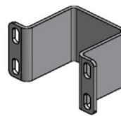
Bowlerhat inkl. rørbøjler 90 x 90 stolpe 691268-03
