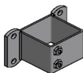
2" frontrør dobbelt inkl. rørbøjler 90 x 90 stolpe 691290-05
